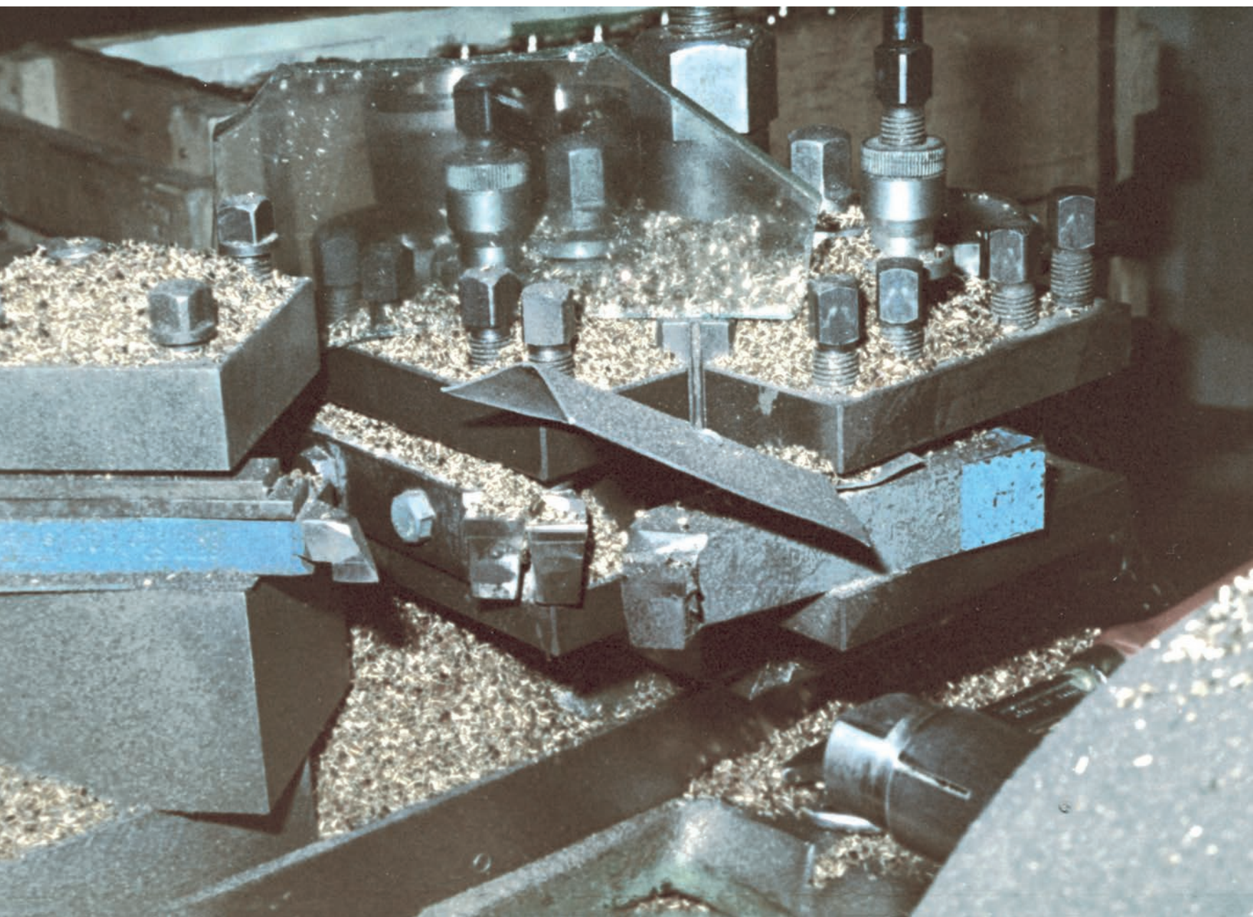
Manuaalisorvin yhden työvaiheen taidokas varta vasten tehty neljän terän teräasetus.
